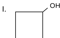
Ciclobutanol
