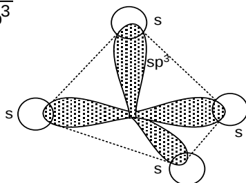
METANO
