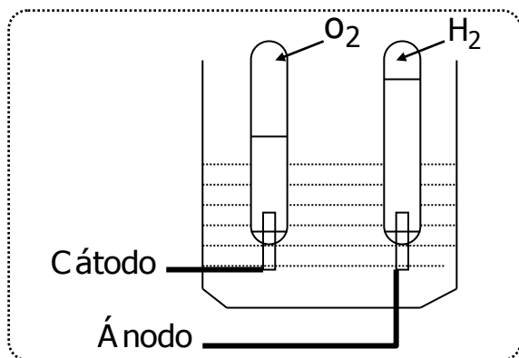
Fig. 10.5 \text{H}_2\text{O} + \text{H}_2\text{SO}_4
