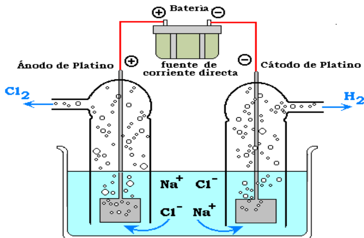
Fig. 10.4 Electrólisis del NaCl acuoso , produciéndose \text{H}_2(\text{g}) en el cátodo y \text{Cl}_2(\text{g}) en el ánodo. Puesto que ambos gases reaccionan explosivamente al ponerse en contacto, deben producirse por separado tal como se muestra en la figura.
