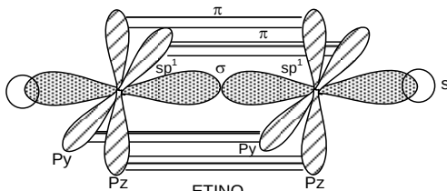
ETINO
